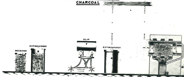
DIAGRAM N°3 APPARATUS FOR BURNING CHARCOAL
